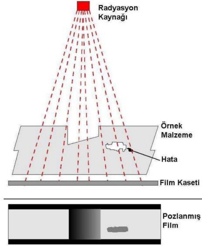
Şekil 17. Radyografik muayenenin çalışma prensibi
