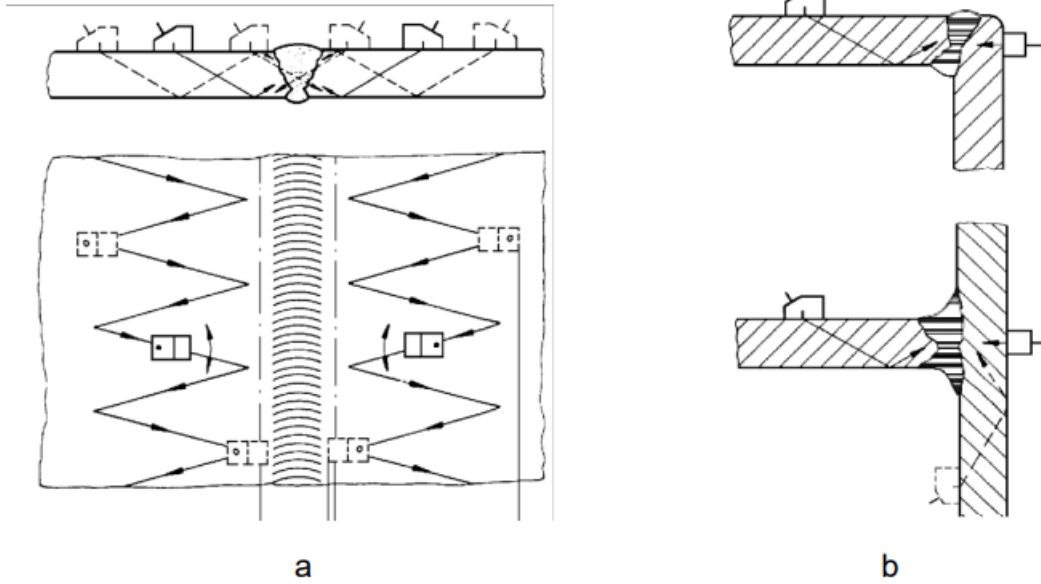
Şekil 15. İncelenen parça üzerindeki prob konumuna göre yansıma şekilleri
