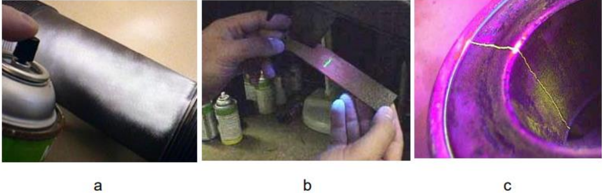
Şekil 3. a) Geliştiricinin uygulanması ve b-c) inceleme
