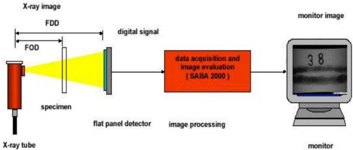
Şekil 19. Radyoskopi yönteminin şematik görünümü
