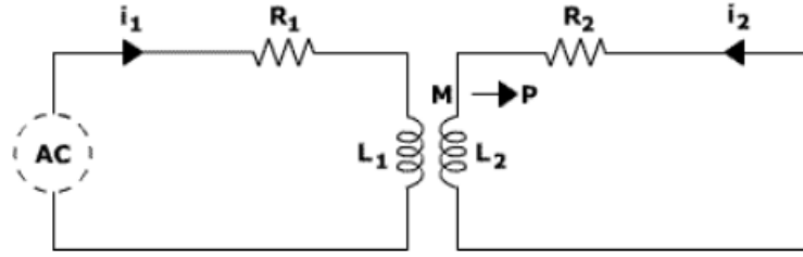
Şekil 4. Girdap akımlarında etkileşim
