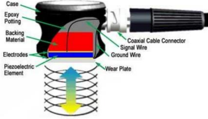
Şekil 12. Tipik bir ultrasonik probun yapısı
