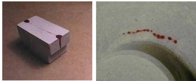
Şekil 1. Penetrant muayene yöntemi uygulanmış iki parça
